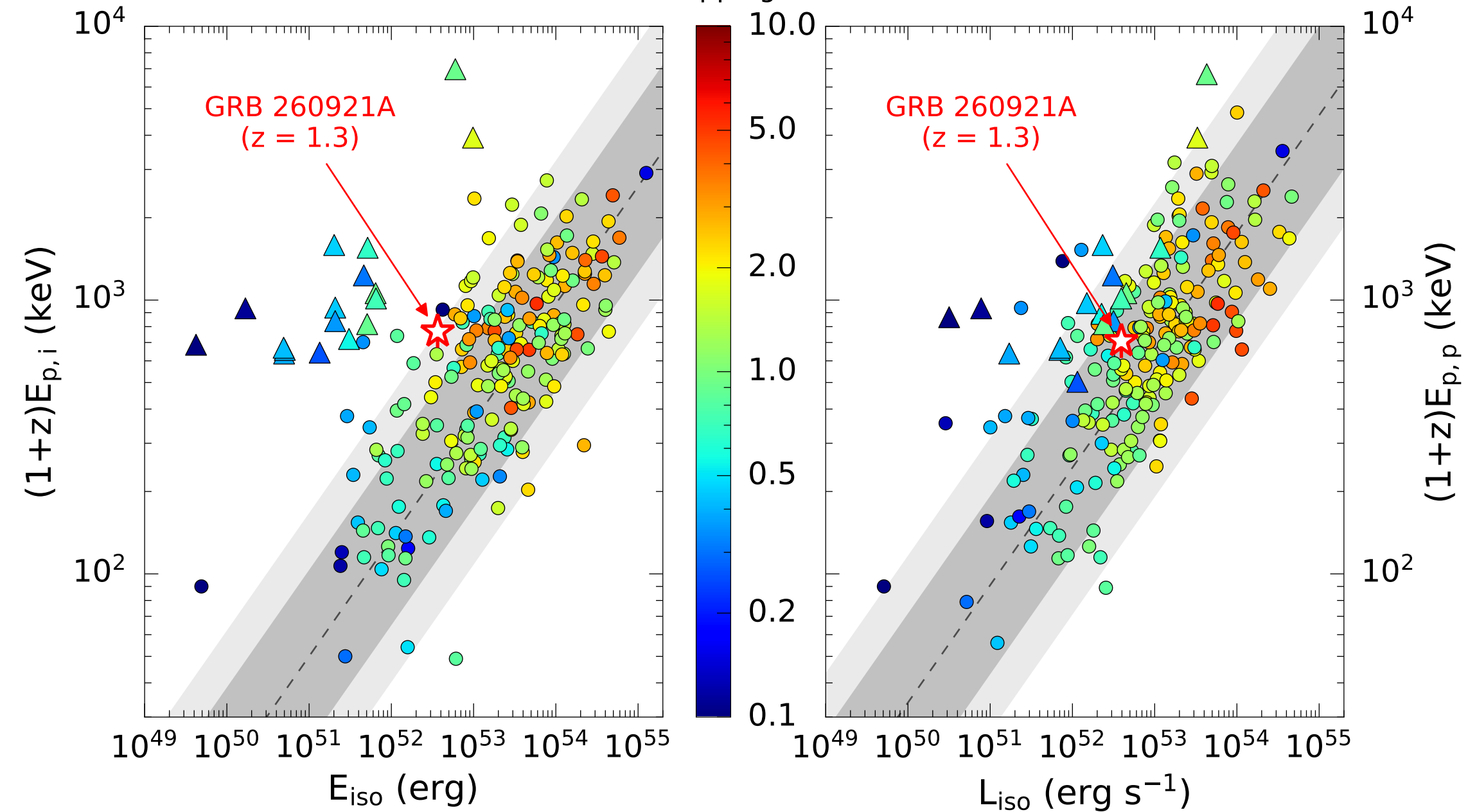
Color mapping: redshift
