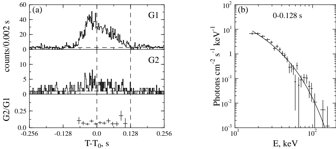
Fig. 3.37.— Burst 980831b.
