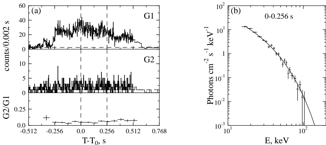
Fig. 3.39.— Burst 980831c.
