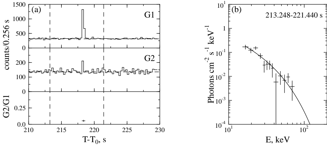
Fig. 3.38.— Burst 980831b (continued).
