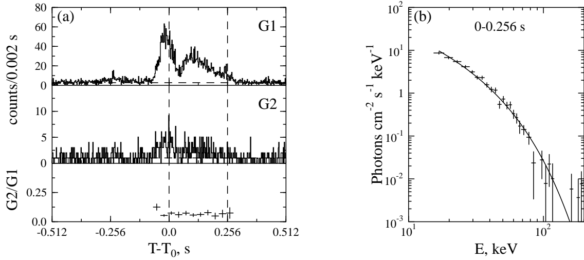
Fig. 3.40.— Burst 980901a.
