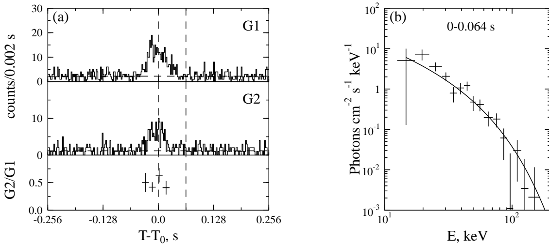
Fig. 4.2.— Burst 961026.
