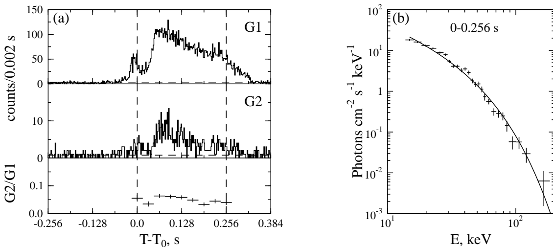
Fig. 4.3.— Burst 961118b (Kosmos 2326).
