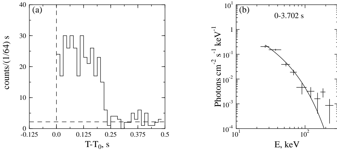
Fig. 4.1.— Burst 790107 (Venera 11).
