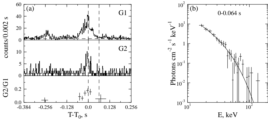
Fig. 5.5.— Burst 980617i.
