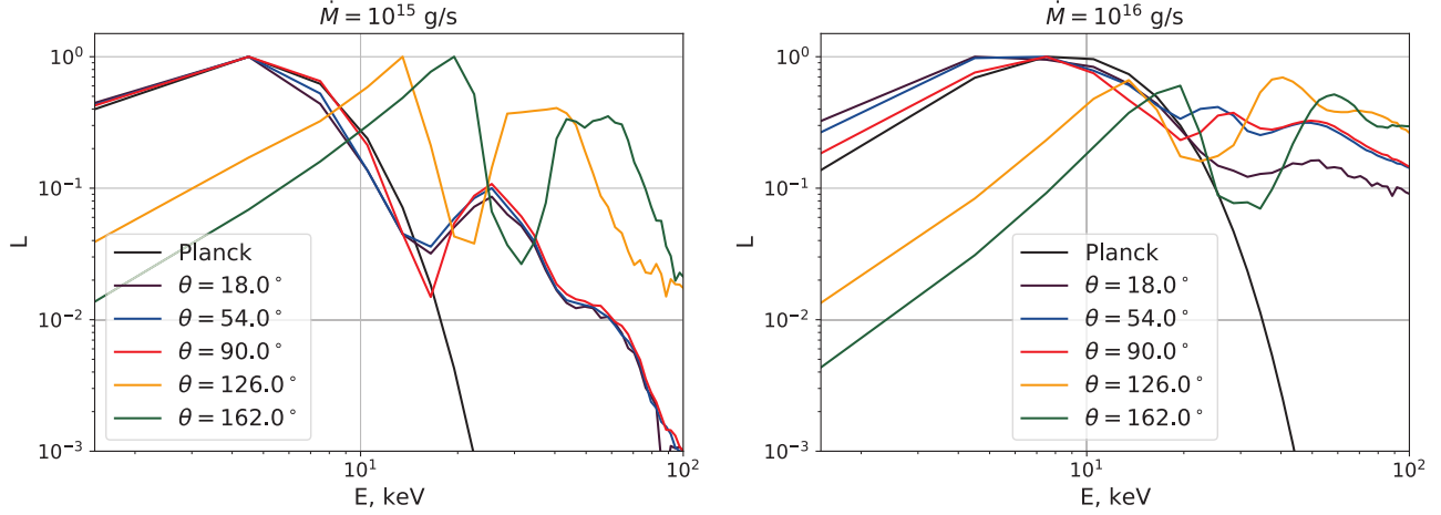
Рис. 1. Зависимость средней по поверхности колонки интенсивности для различных значений угла \theta . Слева темп аккреции \dot{M} = 10^{15} г/с, справа \dot{M} = 10^{16} г/с. Параметры: M = 1.4M_{\odot} , R = 12 км, R_c = 1 км, E_{\text{cyc}} = 20 кэВ
