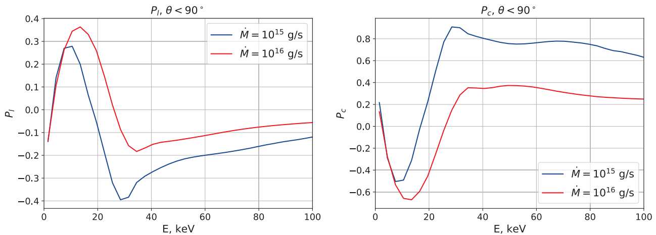
Рис. 2. Слева — степень линейной поляризации в зависимости от энергии фотона, справа — степень круговой поляризации. Результаты усреднены по углам \theta < 90^\circ . Параметры: M = 1.4M_\odot , R = 12 км, R_c = 1 км, E_{\text{cyc}} = 20 кэВ
