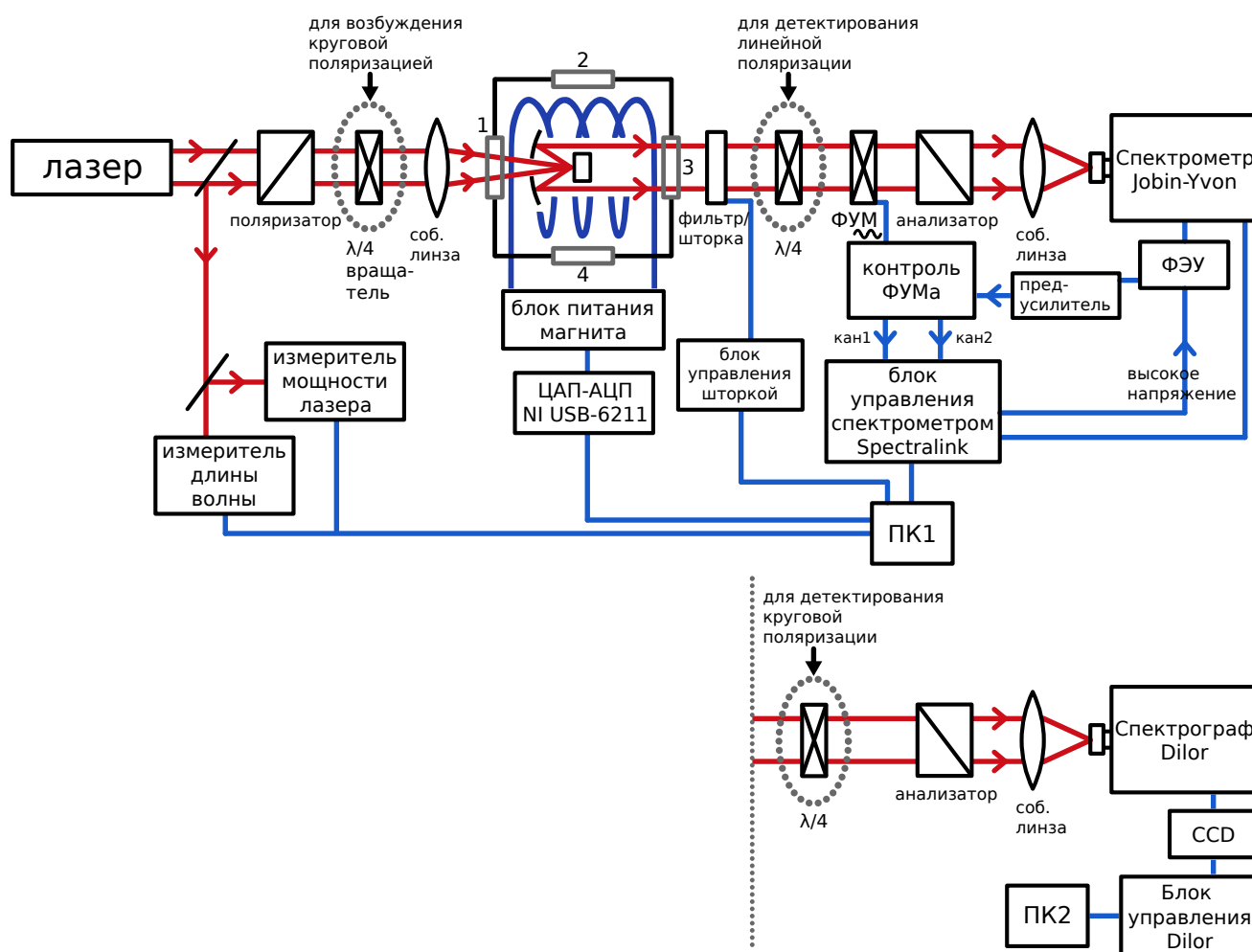
Рис. 1.4: Схема экспериментальной установки. Красным цветом показан ход световых лучей, синим - обмен данными и подача электрического напряжения.
