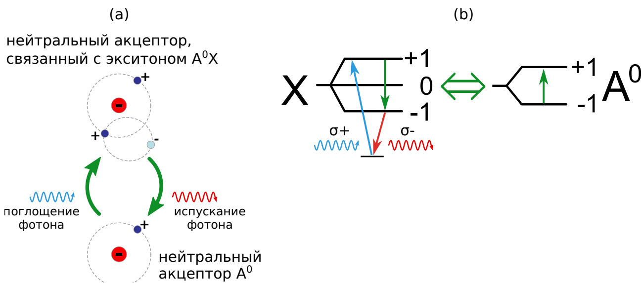
Рис. 1.3: : Неупругое рассеяние света с переворотом спина на нейтральном акцепторе. Зеленая двунаправленная стрелка означает обменное и диполь-дипольное взаимодействие.
