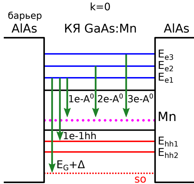
Рис. 4.4: Схема, иллюстрирующая линии переходов между различными подзонами в КЯ GaAs:Mn/AIAs, наблюдаемые в спектре ФЛ на рис. 4.3.
