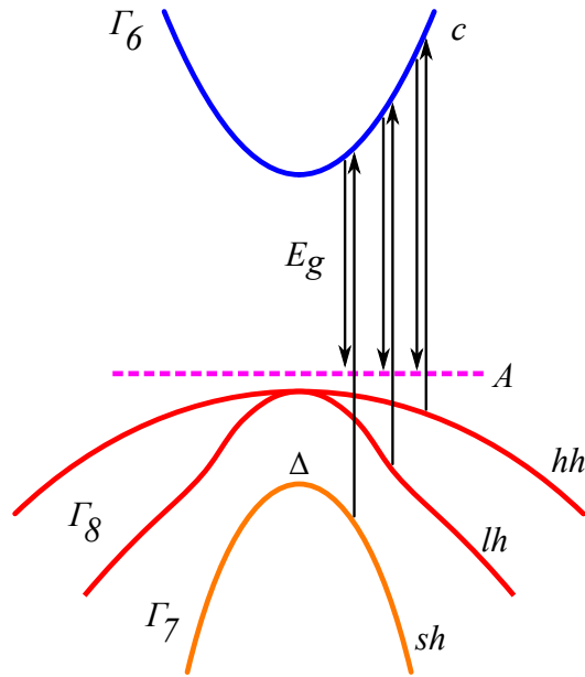
Рис. 1.1: Зонная структура GaAs вблизи центра зоны Бриллюэна и схема переходов на основе рис. из работы [28]. Стрелки, направленные вверх, - возбуждение в зону проводимости ( c ) из подзон тяжелых дырок hh , легких дырок lh и спин-отщепленной sh . Стрелки, направленные вниз, - рекомбинация зона-акцептор ( A ).
