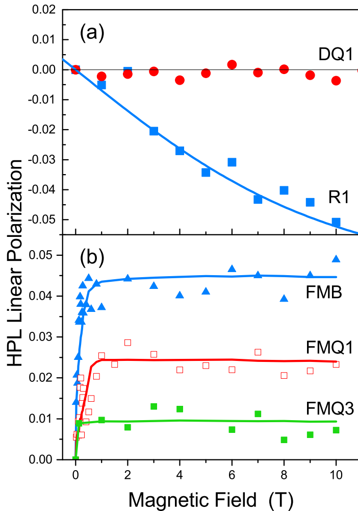
Рис. 4.6: Зависимости степени линейной поляризации ГФЛ от внешнего магнитного поля: (а) измеренная в геометрии Фойгта при температуре T = 5\text{K} для легированных образцов R1 (синие квадраты) и СКЯ DQ1 (красные круги). (b), измеренная в геометрии Фойгта для РМП образцов: FMB (синие треугольники) РМП и СКЯ FMQ1 (красные квадраты) и FMQ3 (зеленые квадраты).
