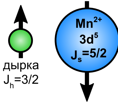
Рис. 3.7: Основное состояние F = 1 комплекса Mn^{2+} + \text{дырка} .
