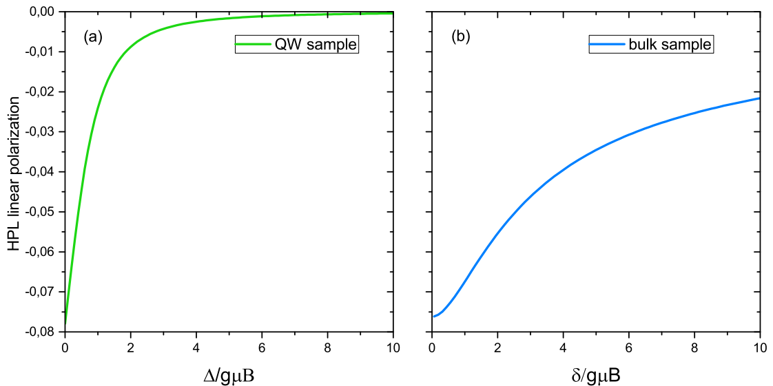
Рис. 4.9: (а) Рассчитанная по формуле (4.7) зависимость линейной поляризации ГФЛ для образца с КЯ от расщепления легкая-тяжелая дырка \Delta , вызванного размерным квантованием, при \delta = 0 . (б) Рассчитанная зависимость линейной поляризации ГФЛ для объемного образца от величины случайных полей \delta , согласно работе [45]. Результаты теоретических расчетов взяты из работы [75].
